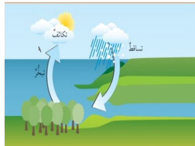
الشكل (8): كيفية حدوث الأمطار الحملية.
