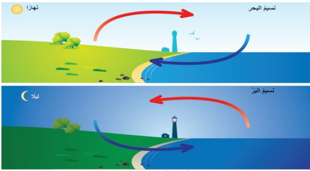
الشكل (5): آلية حدوث نسيم البرّ ونسيم البحر.
