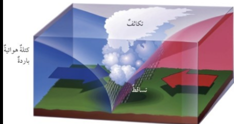
الشكل (9): كيفية حدوث الأمطار الإعصارية.
