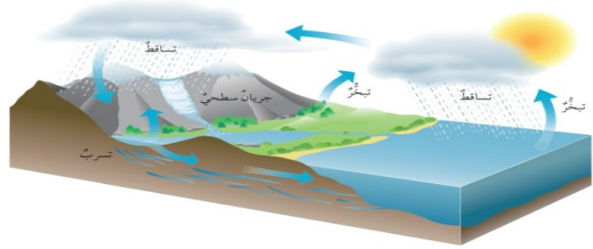
الشكل (6): دورة المياه في الطبيعة.
