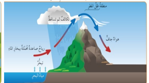
الشكل (7): كيفية حدوث الأمطار التضاريسية.
